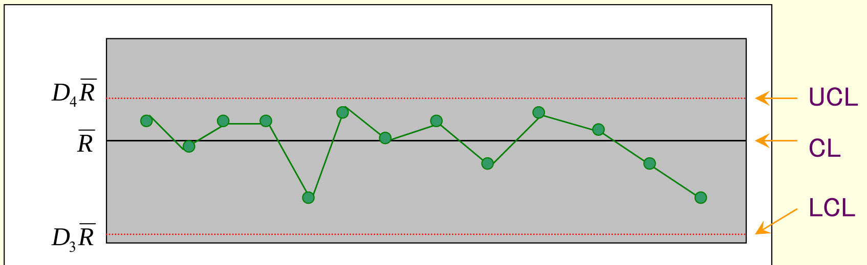
R管理図
