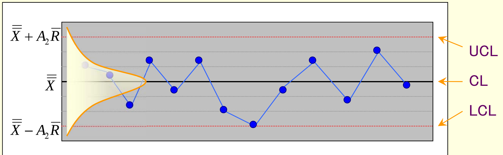
\bar{X} 管理図
