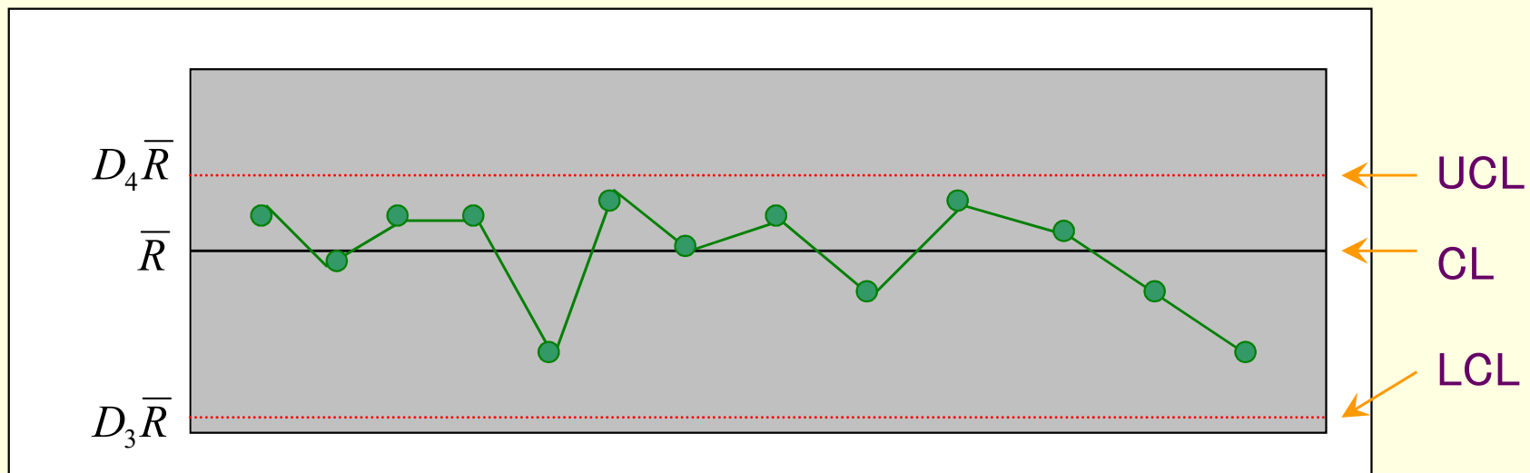
R管理図
