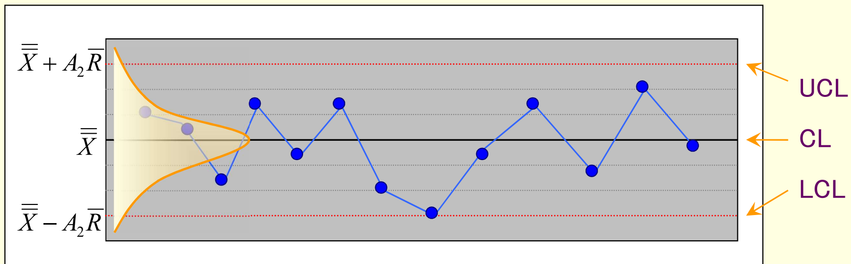
\bar{X} 管理図
