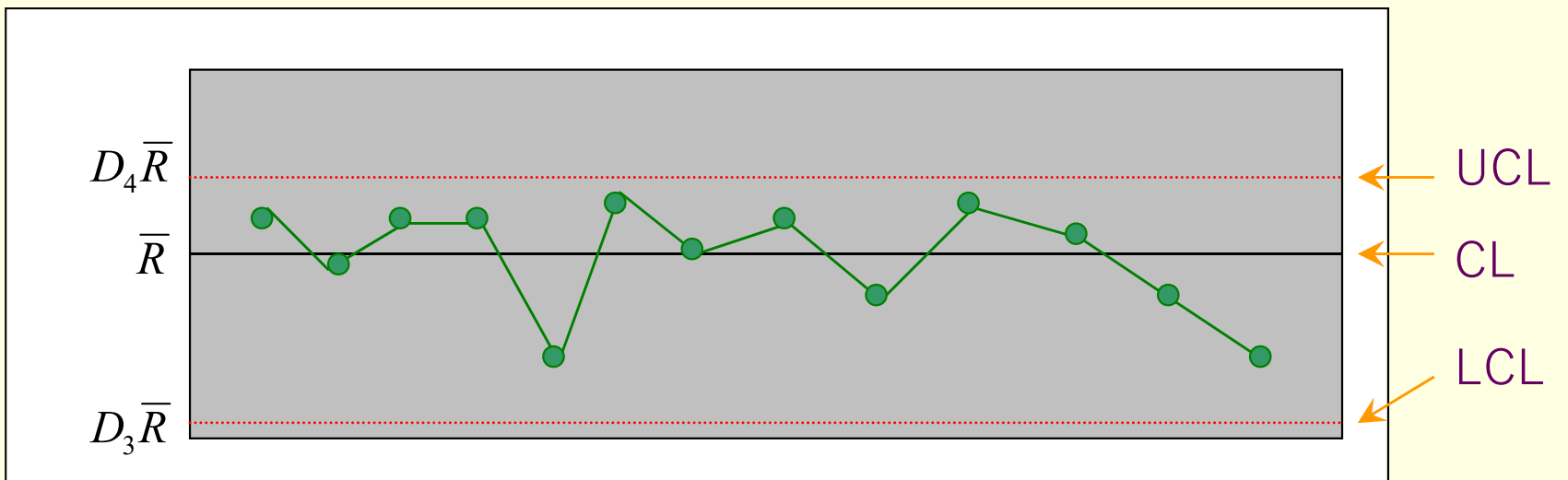
R管理図
