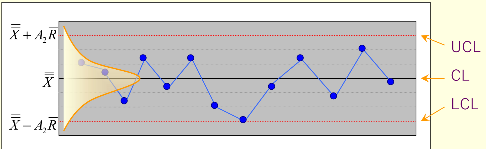
\bar{X} 管理図
