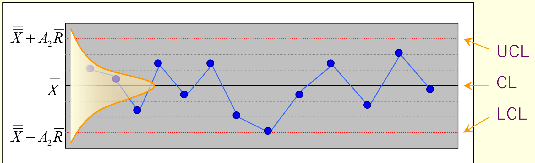
\bar{X} 管理図
