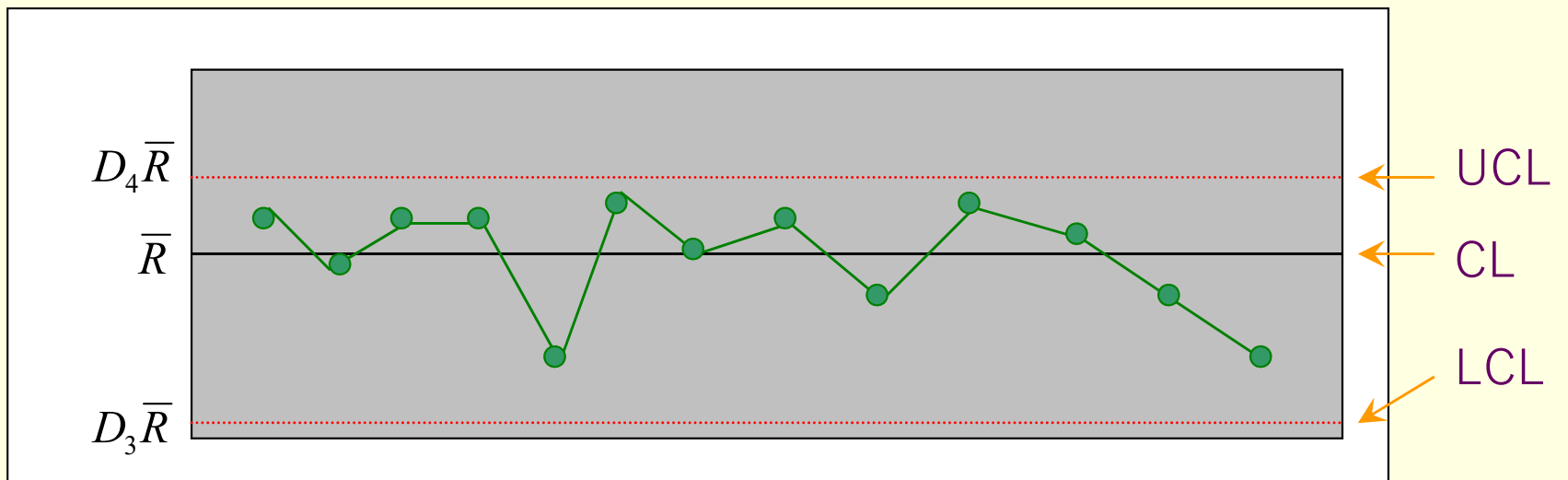
R管理図
