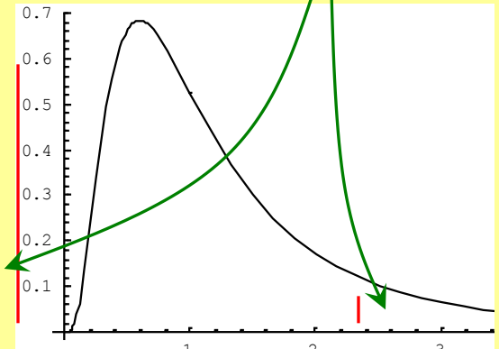
F分布: 両側5%棄却域
